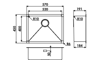
VIBRATO / EVSP54
