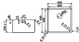
JAVA / EVSP354
