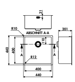
SUPRÊME / EVSP064
