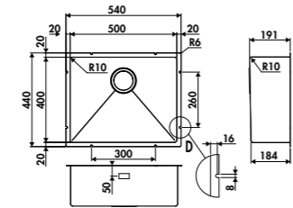
VIBRATO / EVSP57
