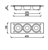
AEGASL10
