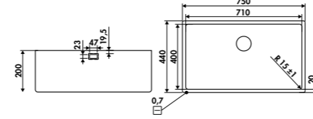
JAVA / EVSP299
